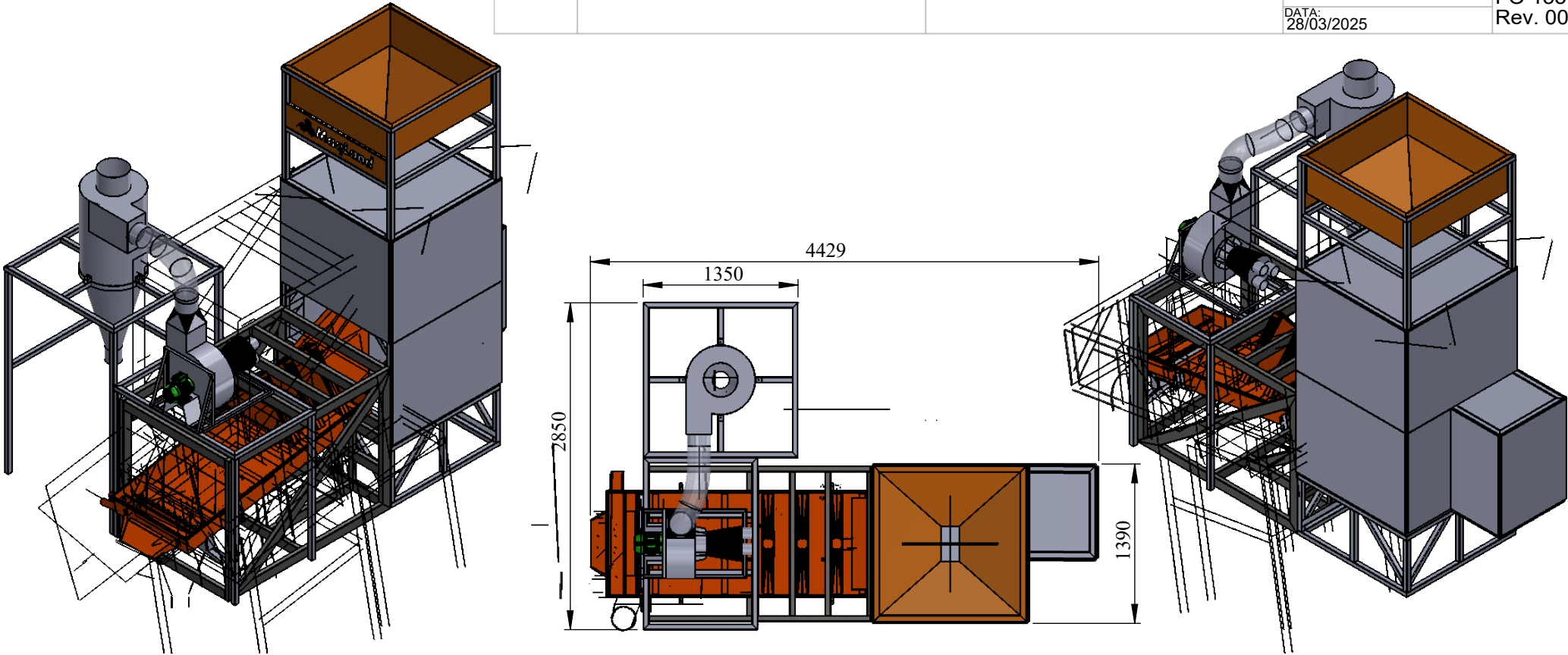
VISTA SUPERIOR
